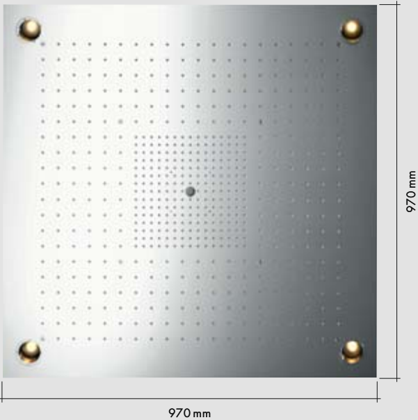
ShowerHeaven 970 x 970 mm mit Licht # 10623800 ShowerHeaven 970 x 970 mm ohne Licht # 10621800 (o. Abb.)
